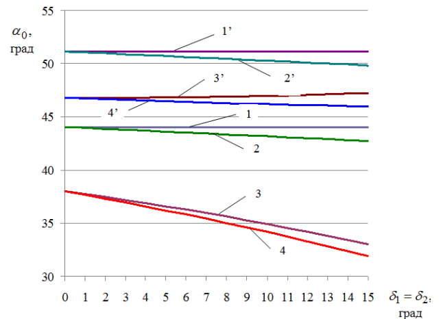
Рис. 2. Графики изменения углов статической устойчивости секций шарнирно-сочлененной машины (' – обозначена задняя секция): 1, 1', 2, 2' – рассчитанные по зависимости \alpha_0 = \arctg(B/2h_c) без учета и с учетом прогиба шин соответственно; 3, 3', 4, 4' – рассчитанные в соответствии с разработанным методом без учета и с учетом прогиба шин соответственно
