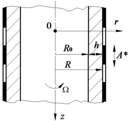
Рис. 1. Розрахункова схема
