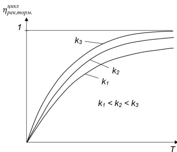
Рис. 1. Зависимость \eta_{\text{рек.торм.}}^{\text{цикл}}(t) .
