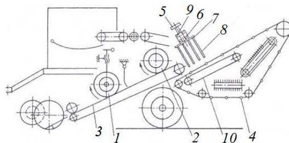
Рис. 1. Схема макетного образца машины для уборки топинамбура
