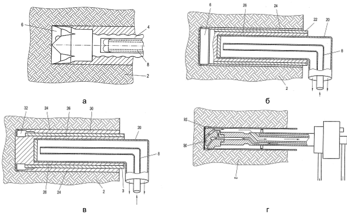
Рис. 16. Теплообмінник: а – передній кінець інженерних засобів з лінією для теплообміну; б, в – варіанти теплообмінного анкера із збільшеною пропускнуною здатністю; г – схема технічних засобів для виготовлення порожнини під теплообмінний анкер
