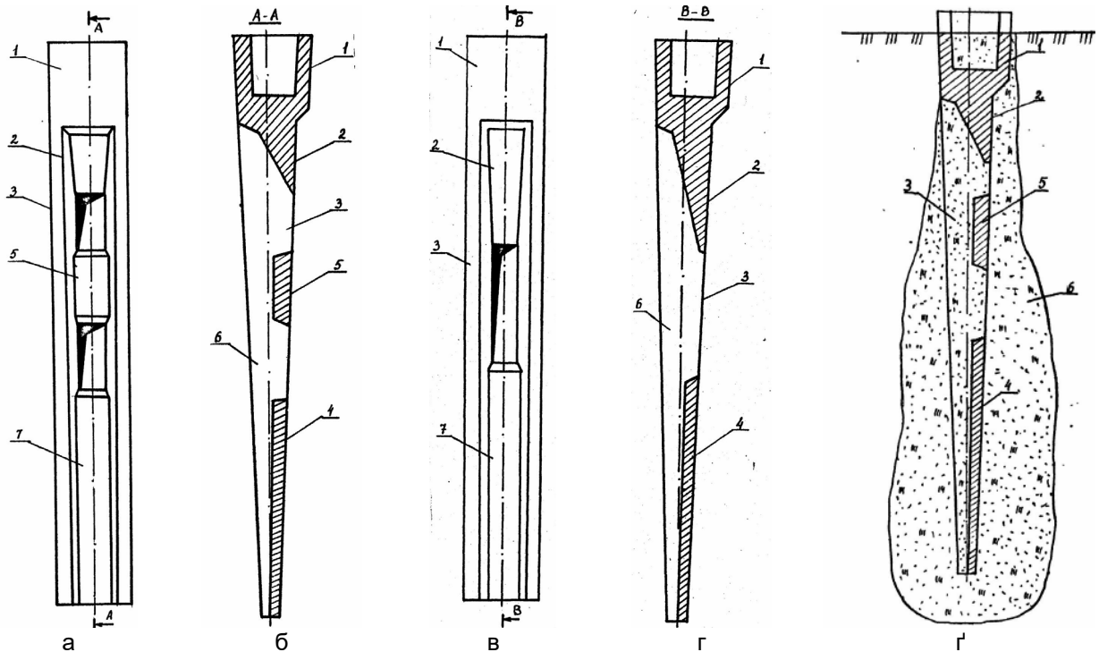
Рис. 11. Палі: а, в – загальний вигляд (варіанти реалізації); б – розріз по А-А на рис. 11.а; г – розріз по Б-Б на рис. 11.в; г' – поздовжній розріз палі, зануреної в ґрунт на проектну глибину
