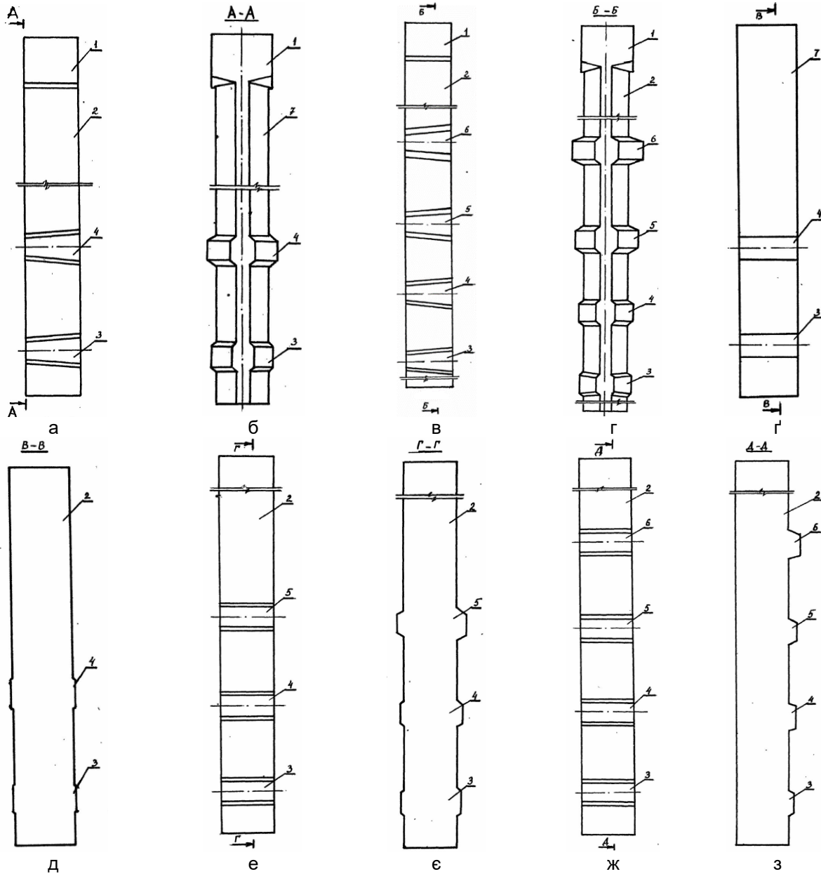
Рис. 10. Забивна паля: а, в, г, е, ж – загальний вигляд (варіанти конструкції); б – вид А-А на рис. 10.а; г – вид Б-Б на рис. 10.в; д – вид В-В на рис. 10.а; е – вид Г-Г на рис. 10.е; з – вид Д-Д на рис. 10.ж
