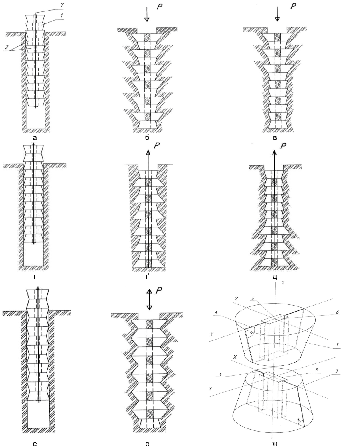
Рис. 8. Палі: а, г, е – конструкція палі в процесі занурення в ґрунт; б, в, г, д, е – конструкція палі в проектному положенні; ж – елементи палі
