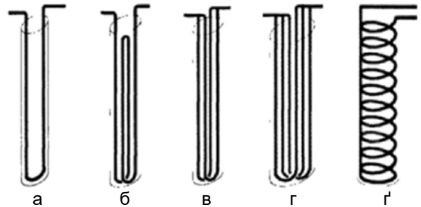
Рис. 2. Принципова схема заглибленої труби різних типів паливового фундаменту: а – одинарні U-подібні труби; б – W-подібні труби; в – паралельні подвійні U-подібні труби; г – паралельні три U-подібні труби; ґ – спіральні труби
