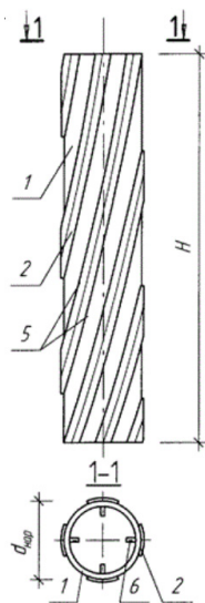
Рис. 17. Гвинтова паля
