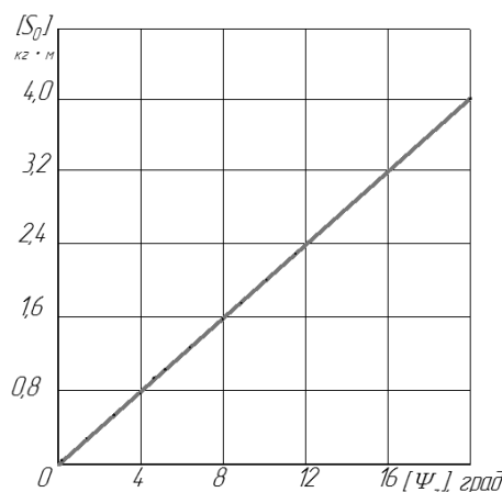
Рисунок 2 – Зависимость максимально-допустимого дисбаланса [S_0] направляющего колеса автомобиля Урал-4320 от максимально-допустимого угла рыскания [\psi_z] .
