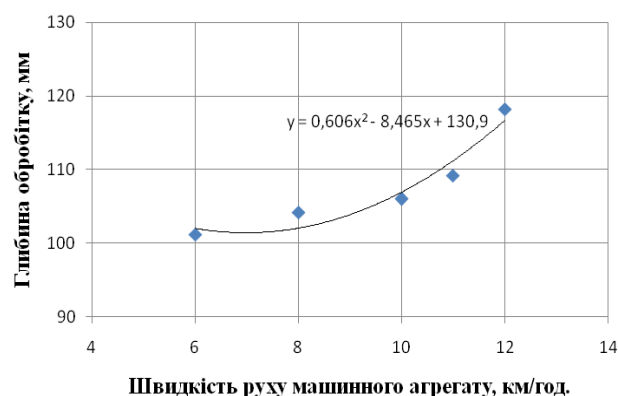
Рис. 8. Зміна глибини дискування при зміні швидкості руху машинного агрегату у складі МТ3-892 + УДА-2,4
