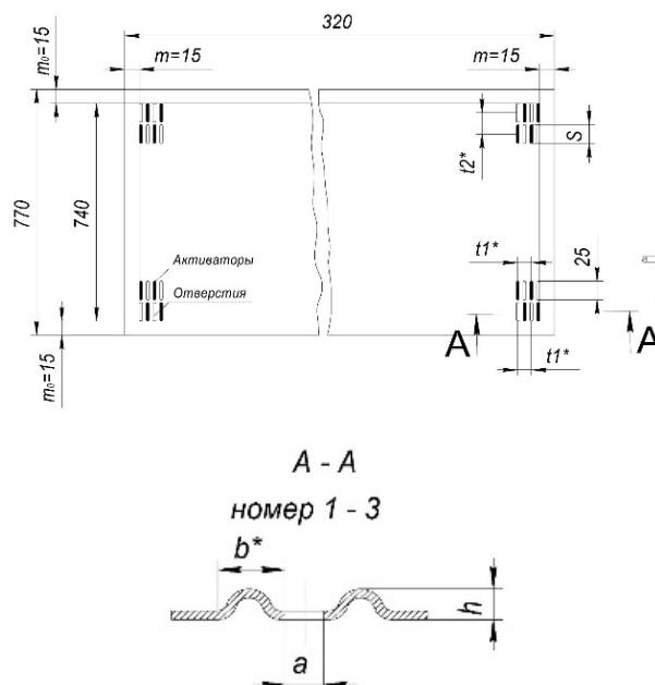
Рис. 7. Креслення розробленого решета з активаторами просіювання
