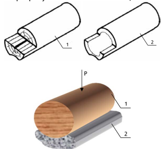
Рис. 5. Схема утворення паливних брикетів з рослинних відходів з різними деформаційними властивостями 1-тверді частини; 2-пластичні частини
