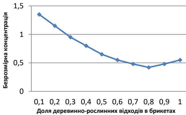
Рис. 9. Залежність безрозмірної концентрації небезпечних викидів від доли деревинно-рослинних відходів в брикетах
