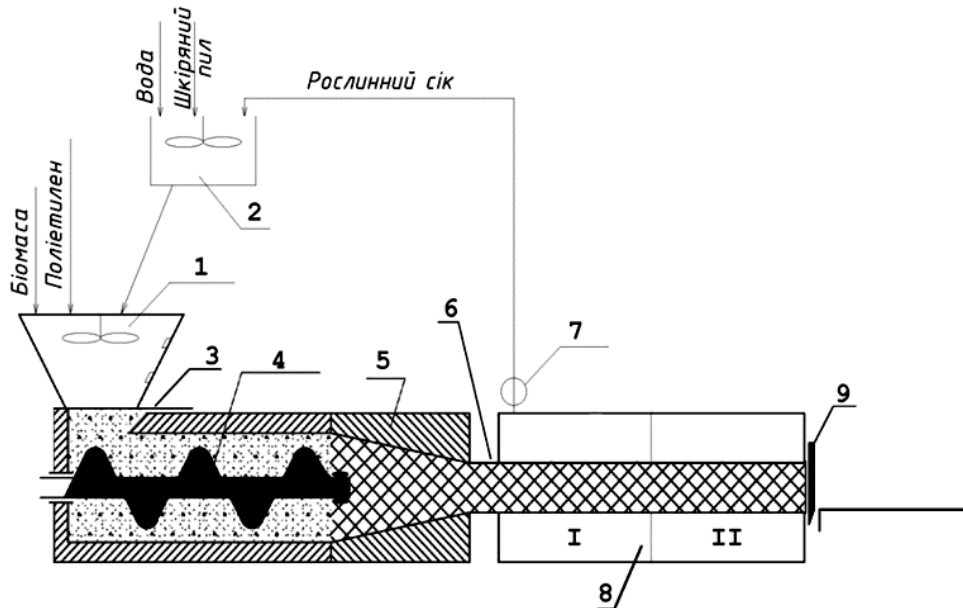
Рис. 8. Прес-автомат гнучкої технології виробництва паливних брикетів: I - перша секція мікрохвильового пристрою на основі системи хвилевідного типу має довжину l_1 ; II – друга секція мікрохвильового пристрою (адаптер) на основі уповільнюючої системи довжиною l_2 ; 1-змішувач брикетної суміші; 2 – змішувач тиксотропної добавки; 3 – засувка; 4 – шнековий транспортер; 5 – формуюча головка; 6 – тefлонова труба з отворами; 7 – насос; 8 – камера термообробки НВЧ типу; 9 – ніж та стіл для охолодження брикетів.
